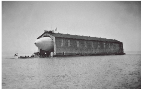
Motiv im Juni: LZ 1 bereit zur Ausfahrt aus der schwimmenden Halle. Die Heckspitze des Luftschiffs ragt aus der Toröffnung.
